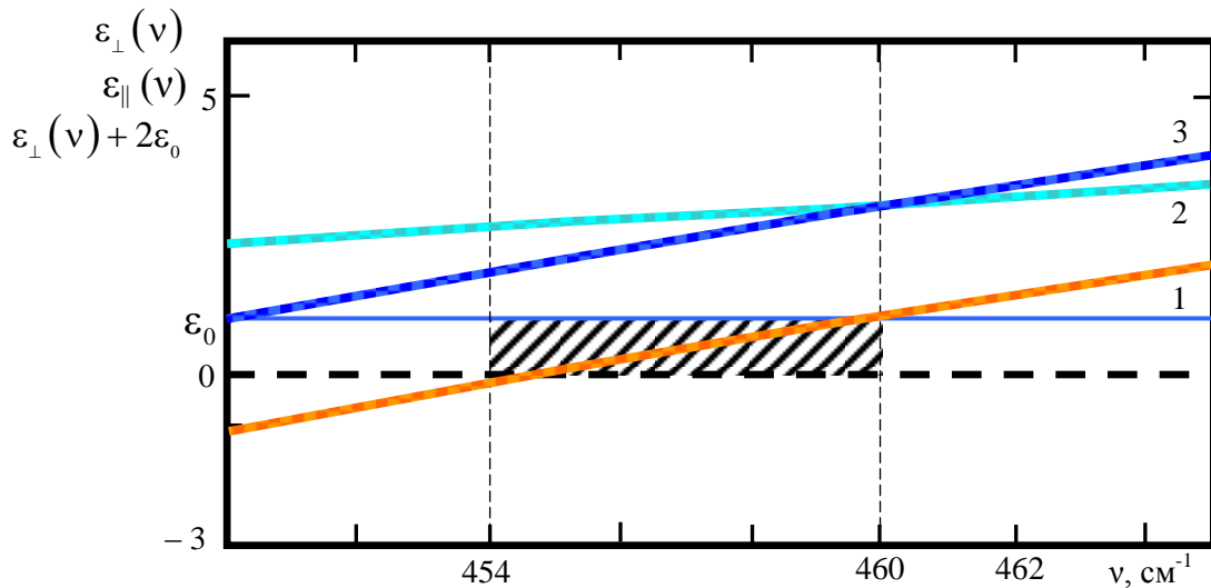
Рис. 2. Залежність дійсної частини діелектричної проникності від частоти в діапазоні існування СПП згідно умов (4): 1 – \epsilon_{\perp}(v) ; 2 – \epsilon_{\parallel}(v) ; 3 – \epsilon_{\perp}(v) + 2\epsilon_0 .
