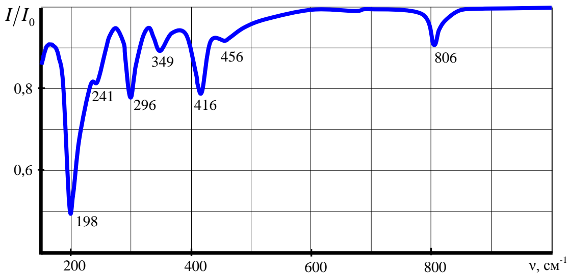
Рис. 4. Розрахункові спектри ППВВ \text{LiNbO}_3 при орієнтації C \parallel x .
