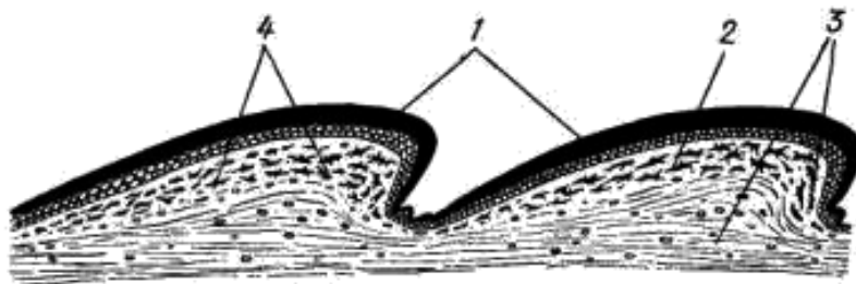
Рис. 68. Схема поперечного розрізу шкіри ящірки:
