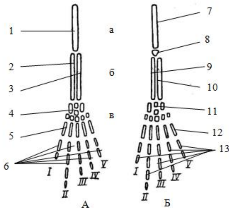
Рис. 50. Схема будови парних кінцівок наземних хребетних:
