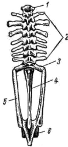
Рис. 47. Осьовий посткраніальний скелет та тазовий пояс жаби (вигляд згори):
